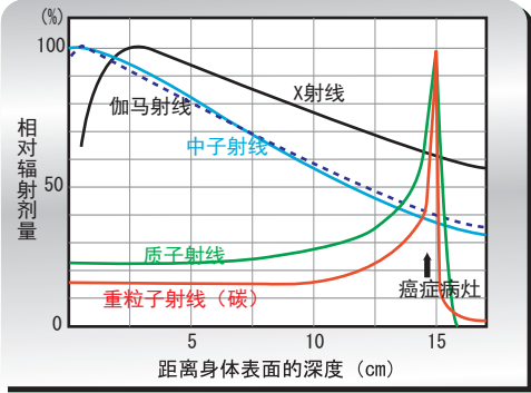
各种放射线在生物体内的辐射剂量分布
